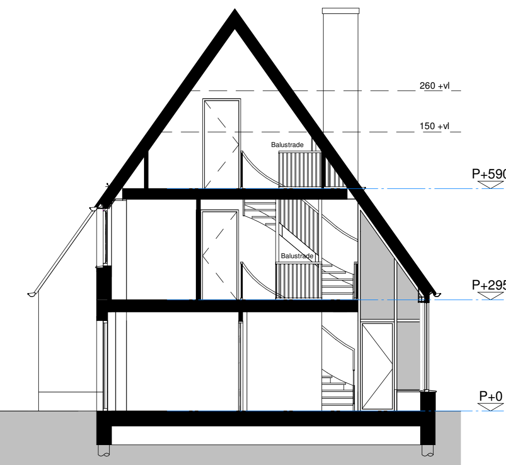
Doorsnede BB 1:100
