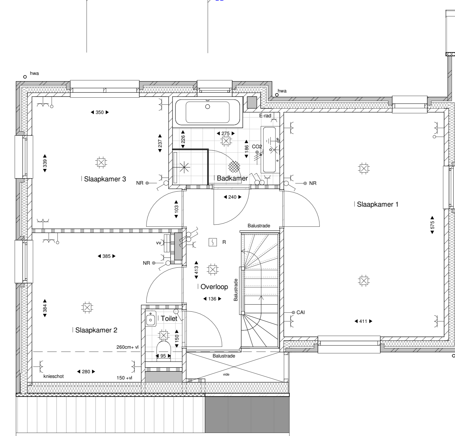
Tweede verdieping 1:100
