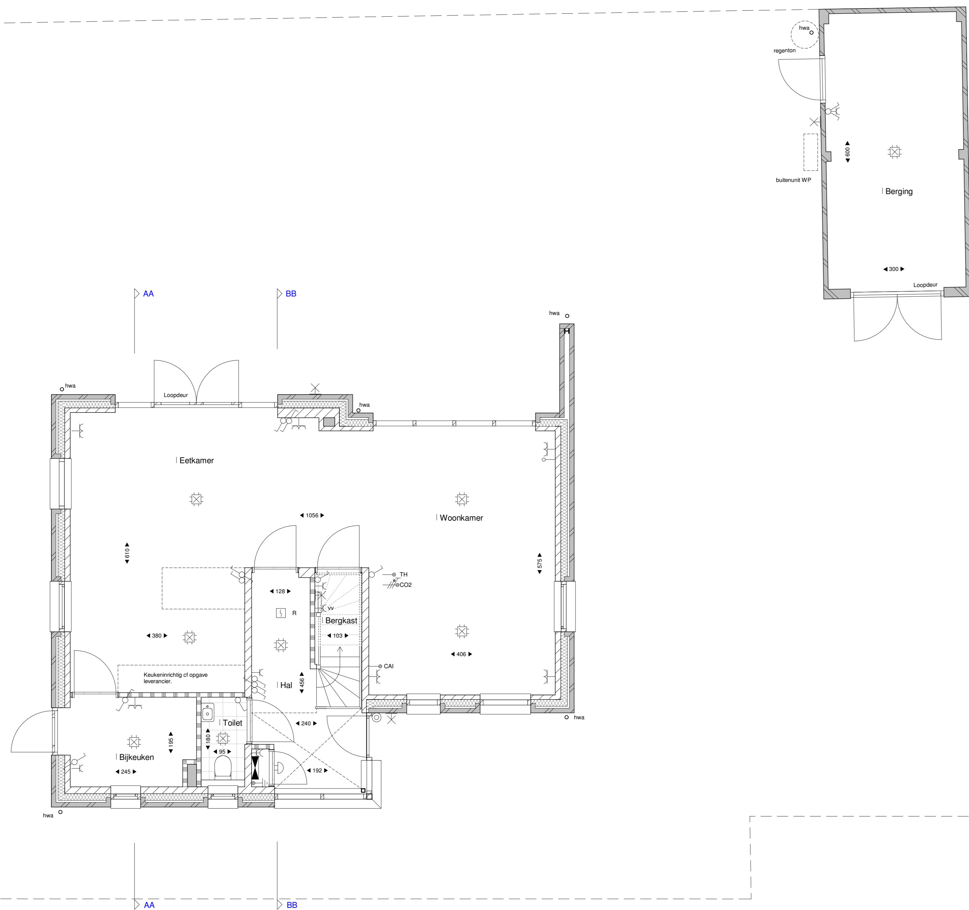
Begane grond 1:100
