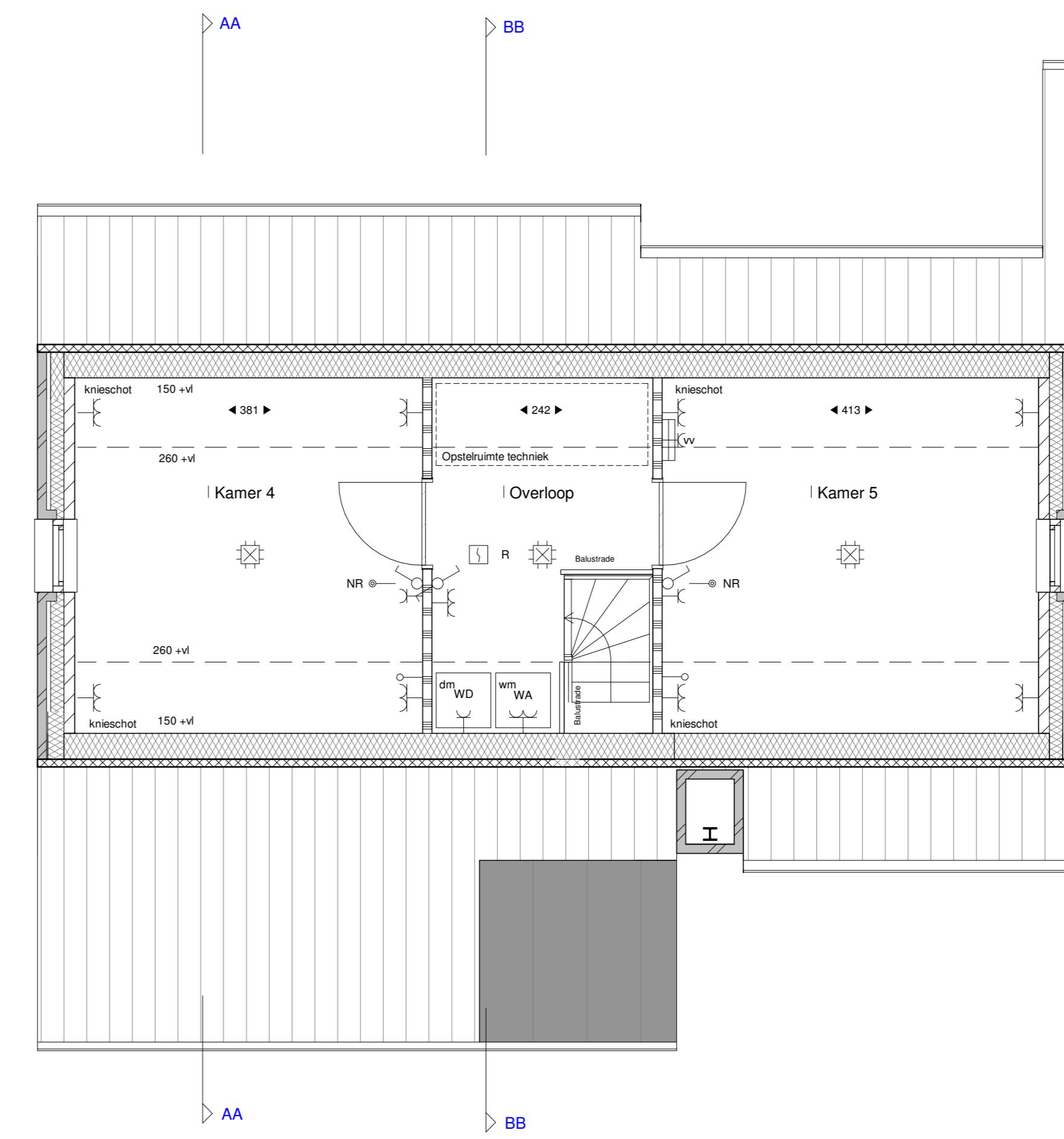
Tweede verdieping 1:100
