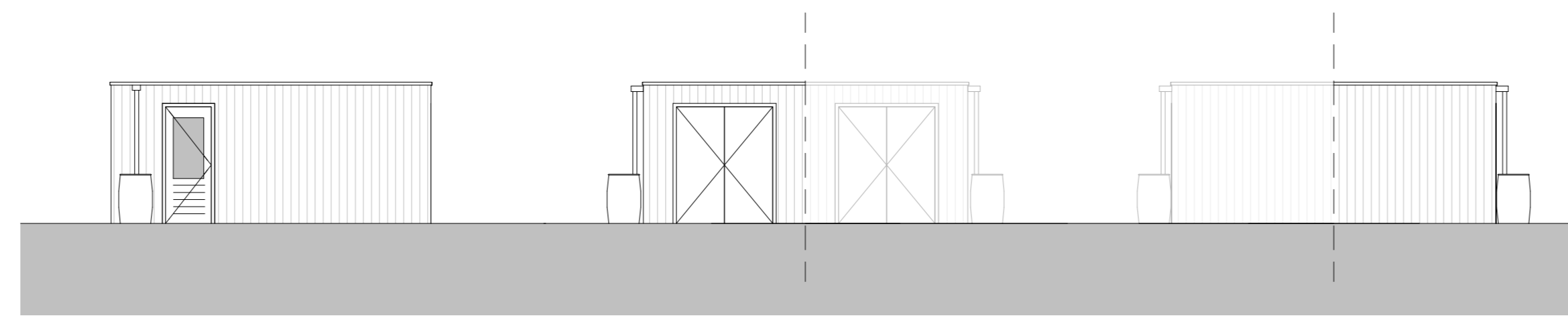
Linkerzijgevel 1:100
