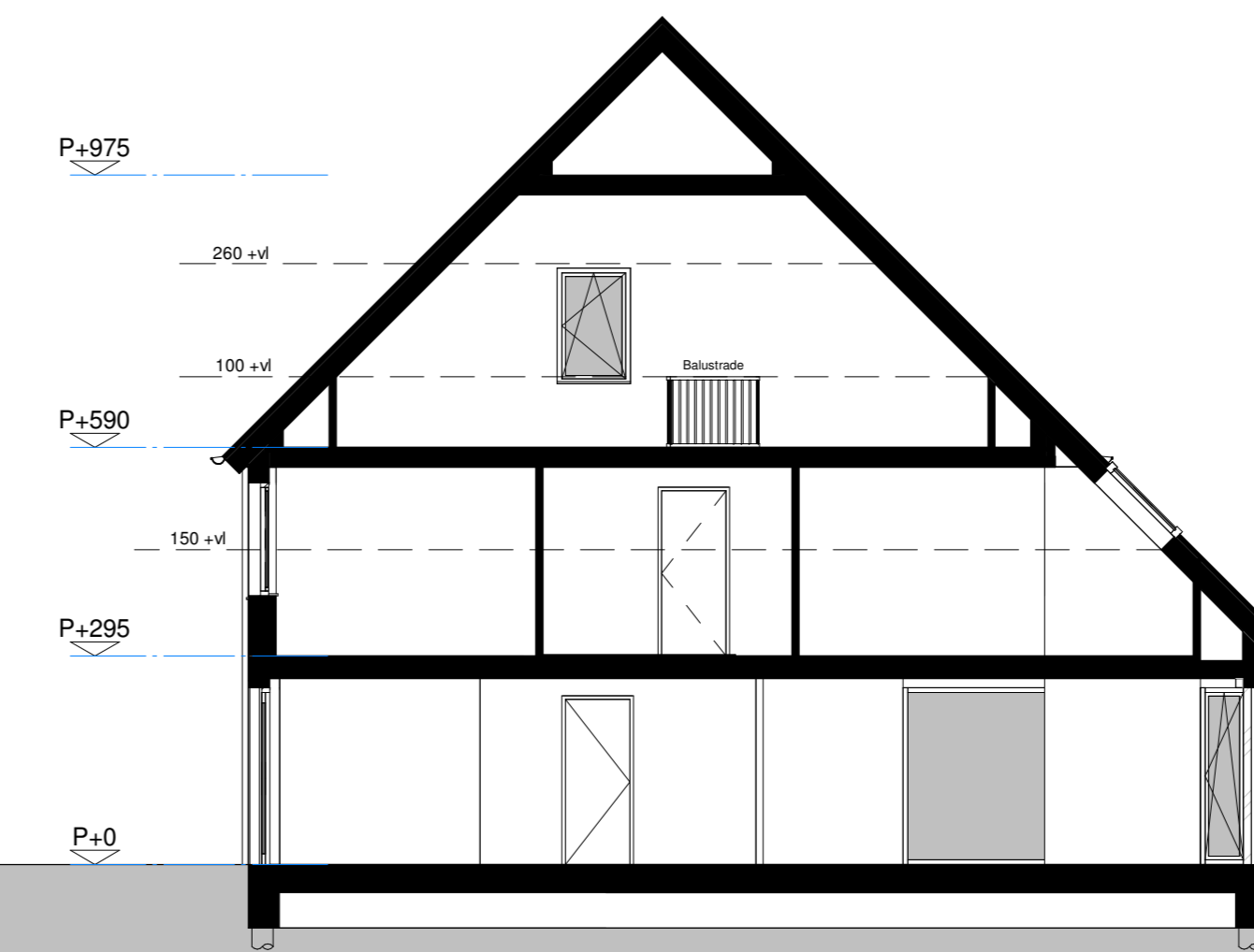
Doorsnede BB 1:100
