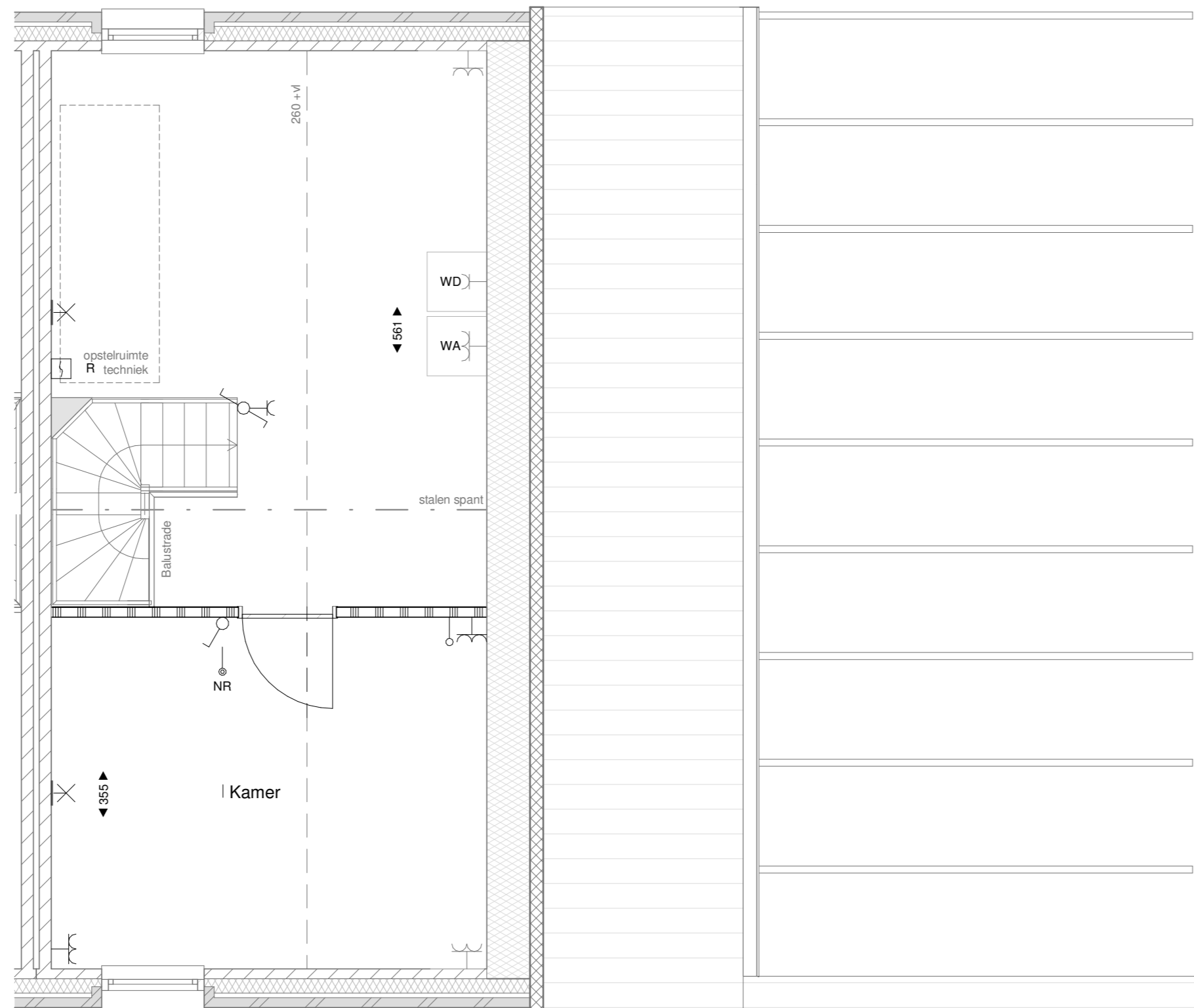
Tweede verdieping 1:50
