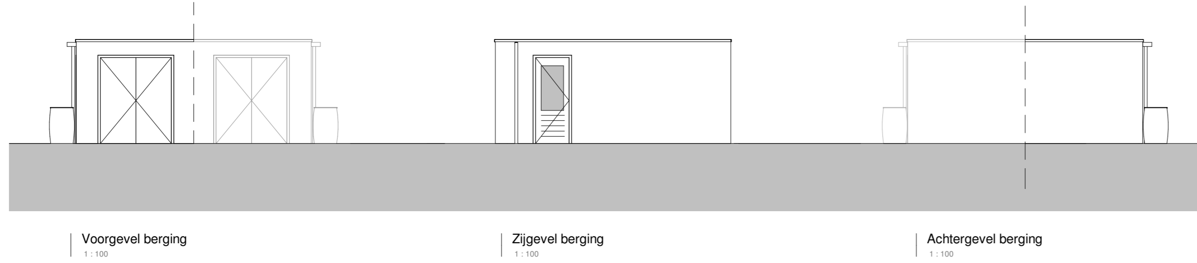
Voorgevel berging 1:100
