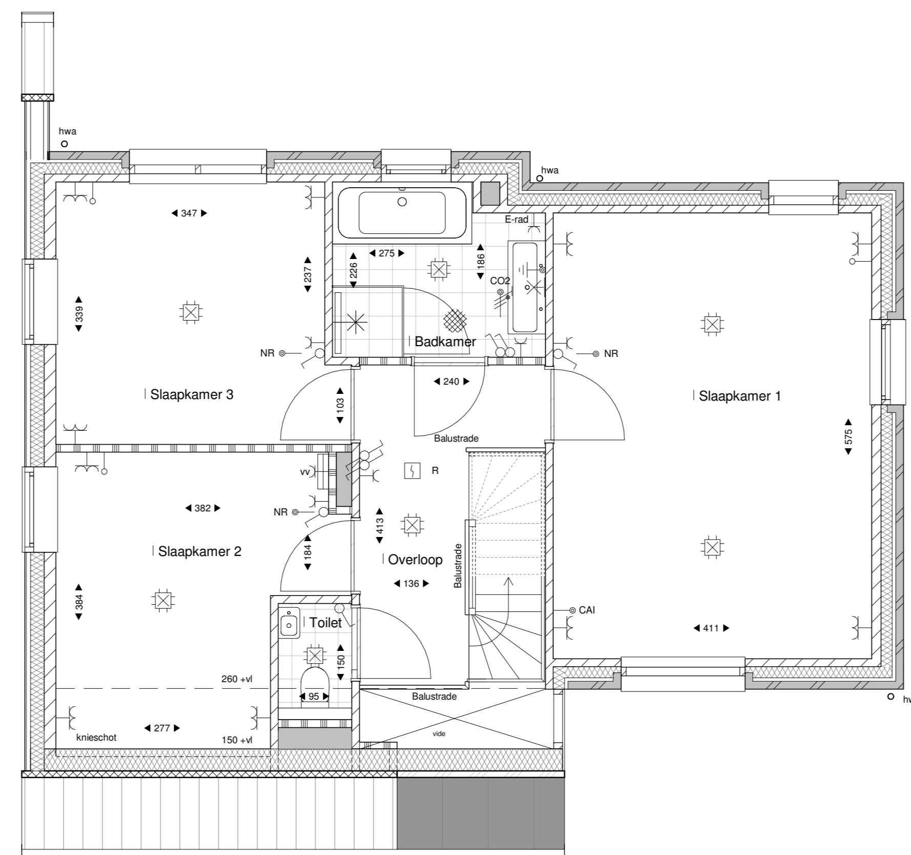
Eerste verdieping 1:100
