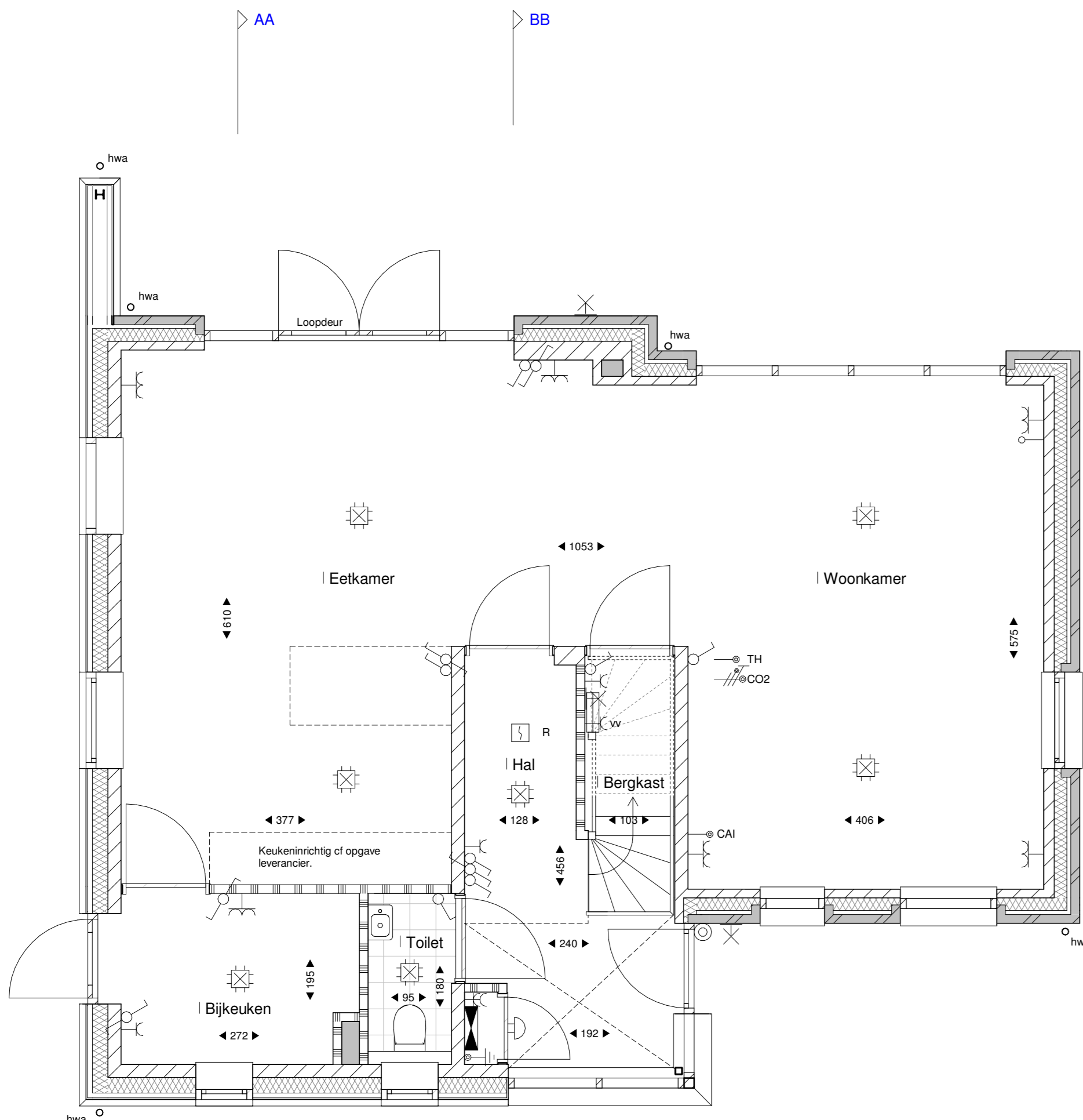
Begane grond 1:100
