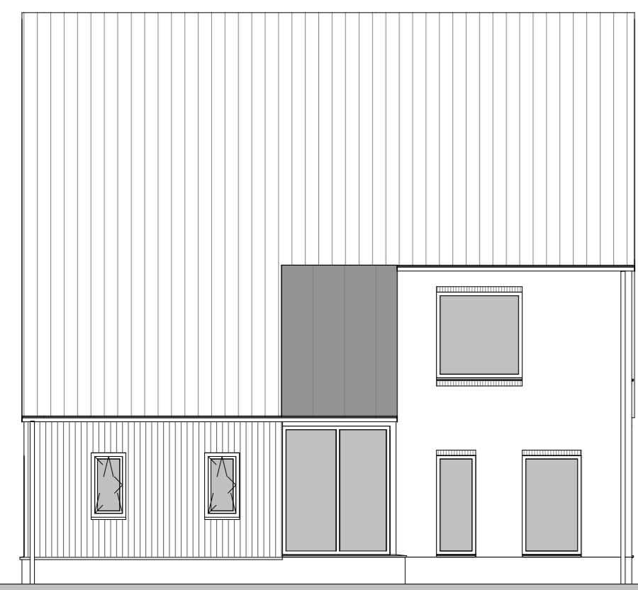
Voorgevel 1:100
