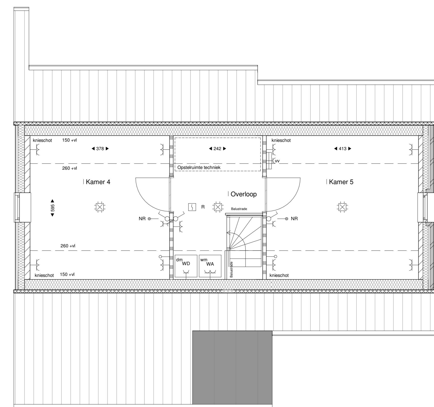
Tweede verdieping 1:100
