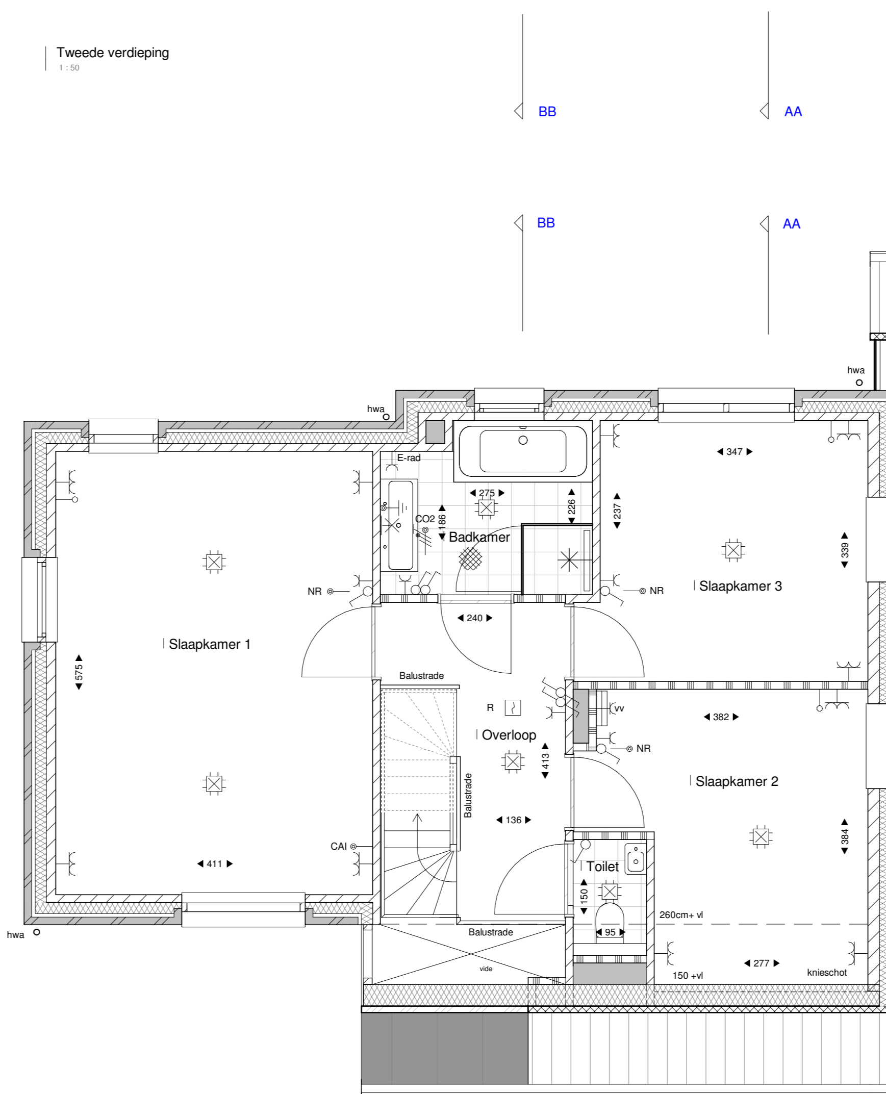
Eerste verdieping 1:100
