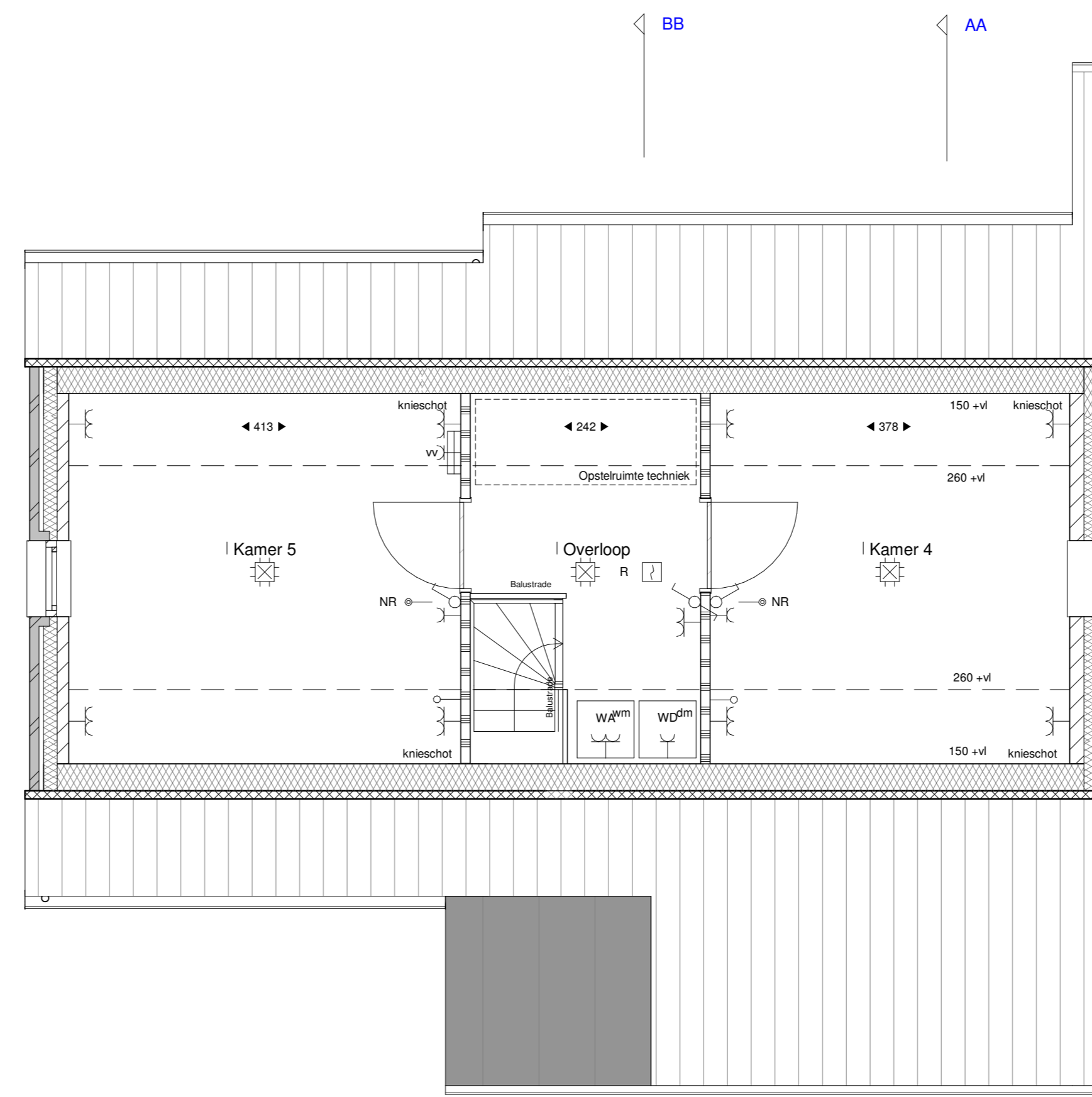
Tweede verdieping 1:100
