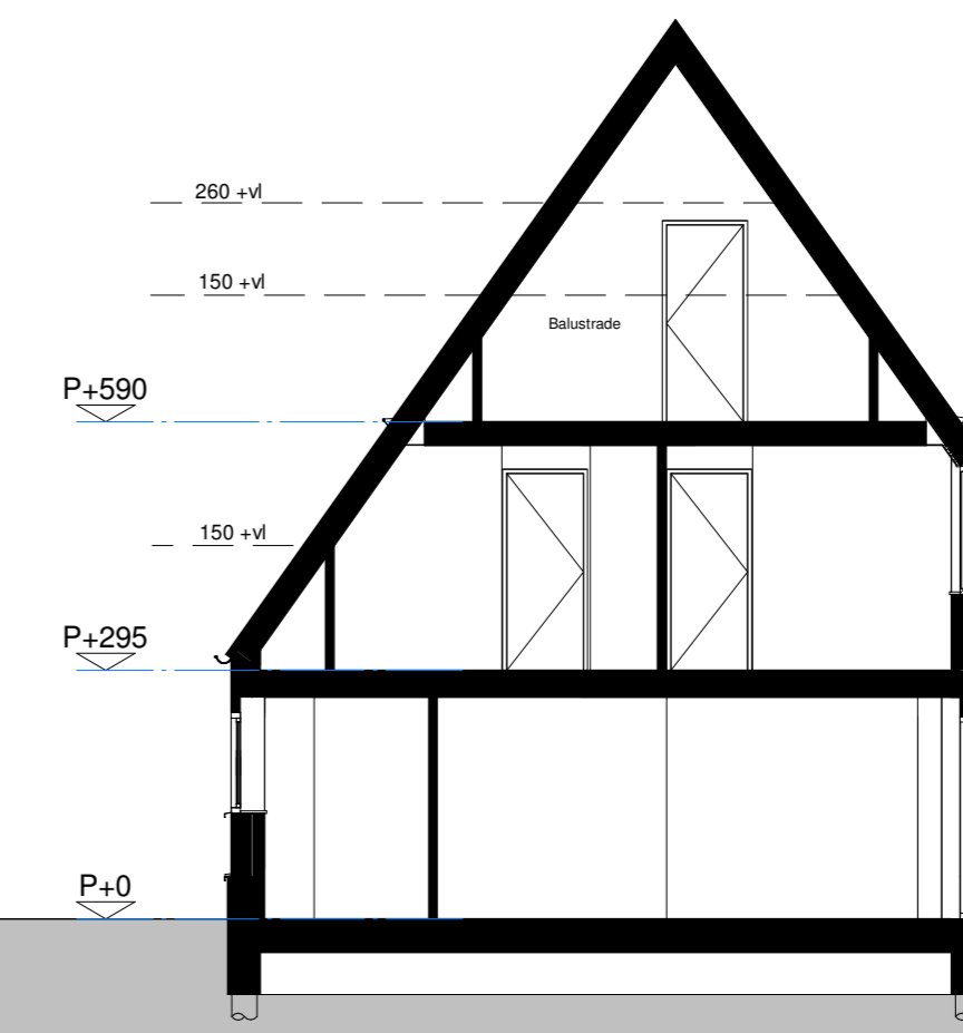
Doorsnede AA 1:100
