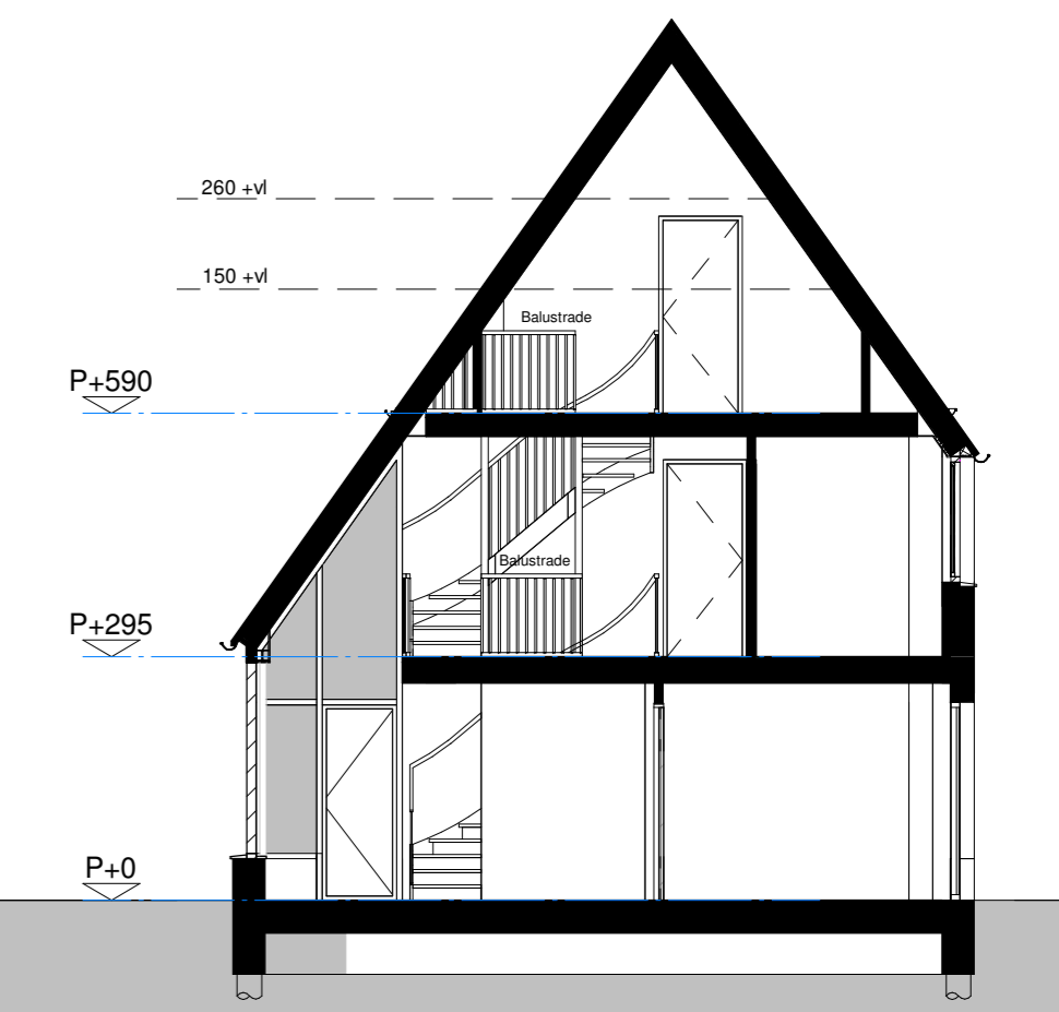
Doorsnede BB 1:100
