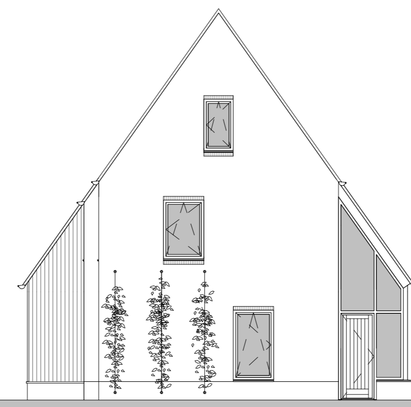
Linkerzijgevel 1:100
