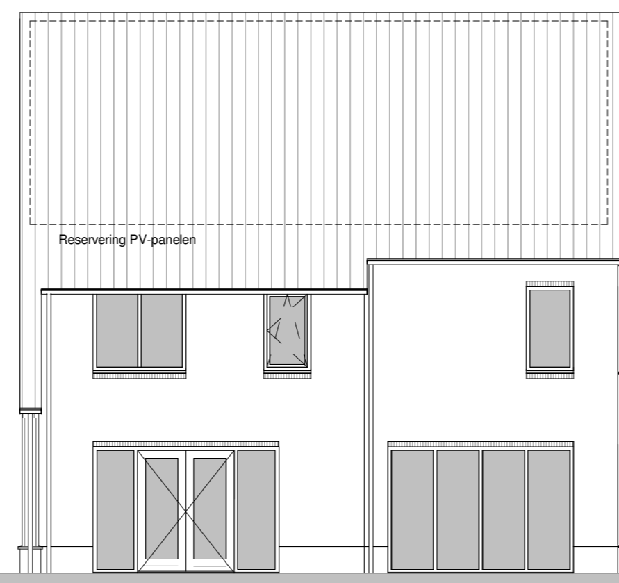
Achtergevel 1:100
