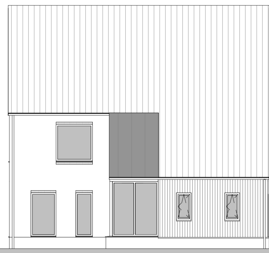
Voorgevel 1:100
